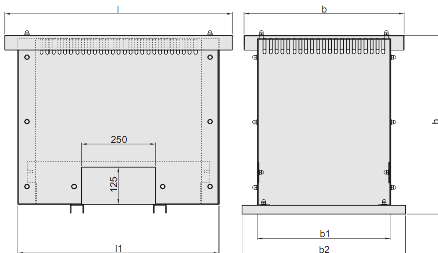
Fig. 2 Golvskap
